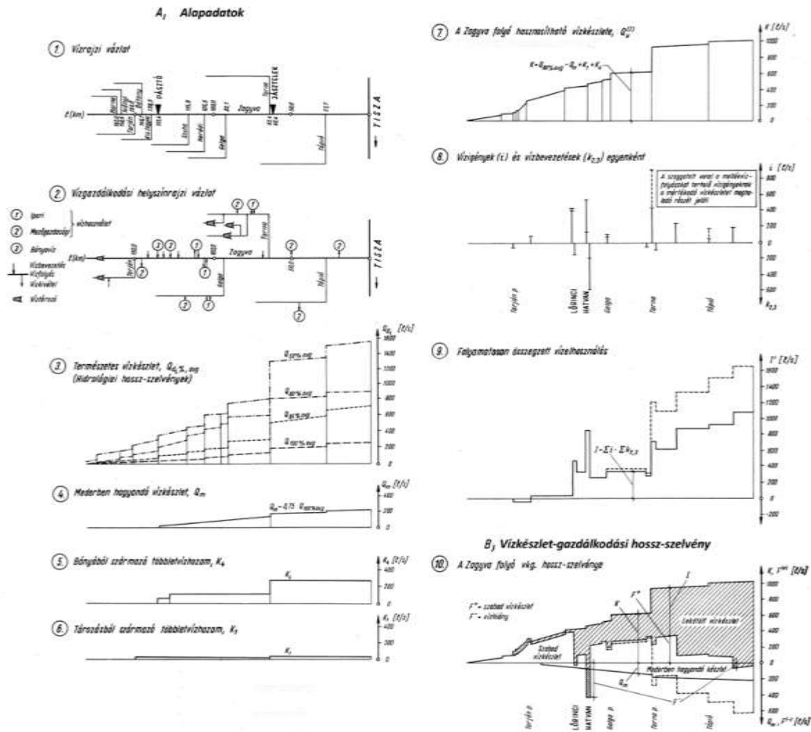
Figure 5: Step-by-step explanation of the longitudinal water balance profile plot (based on: Bözsöny Dénes - Domokos Miklós: Gyakorlati vízkészletgazdálkodás (Tankönyvkiadó, Budapest, 1975)
